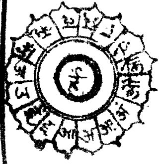
नाभिमंडल
